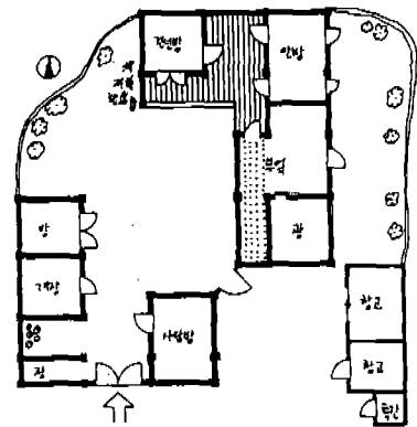
<도면 2> 정언년 할머니댁 평면도 (호주 : 안완균, 1995)
