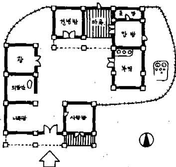
〈도면 7〉 정귀녀 할머니댁 평면도(1945)
