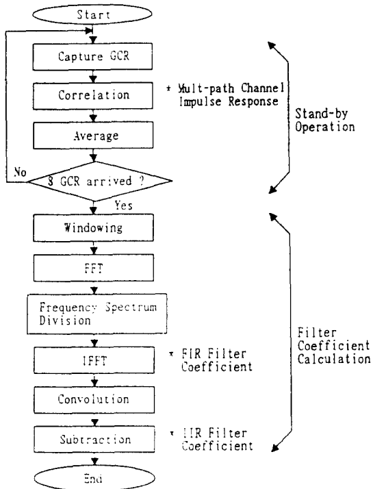
그림 8. 고스트 제거 필터 계수 연산과정 Fig. 8 The calculation process of ghost cancellation filter coefficient
