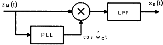
그림 5. 동기 검파기 Fig. 5 Synchronous Detector
