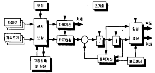
〈그림 1〉 스트랩다운 관성항법장치
