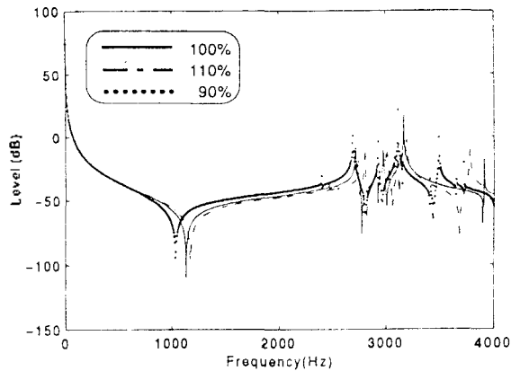
그림 8. 강성 변경에 따른 주파수 응답 함수의 비교
