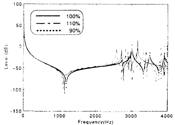
그림 9. 질량 변경에 따른 주파수 응답 함수의 비교
