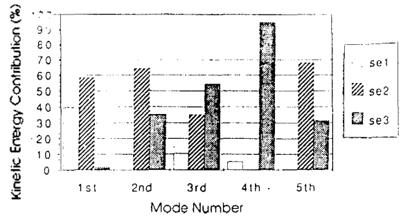
그림 7. 각 요소의 운동 에너지 기여도
