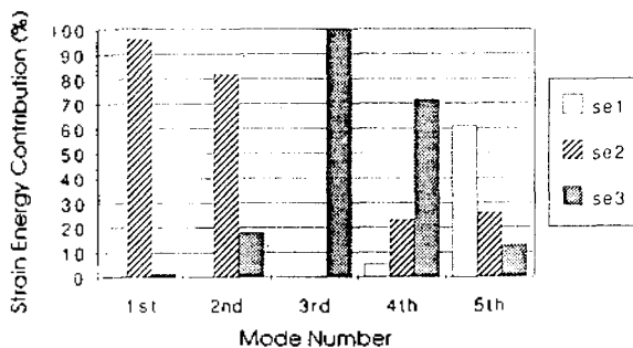
그림 6. 각 요소의 변형 에너지 기여도
