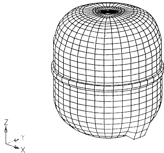
그림 4. 컴프레서 셀의 유한 요소 모델
