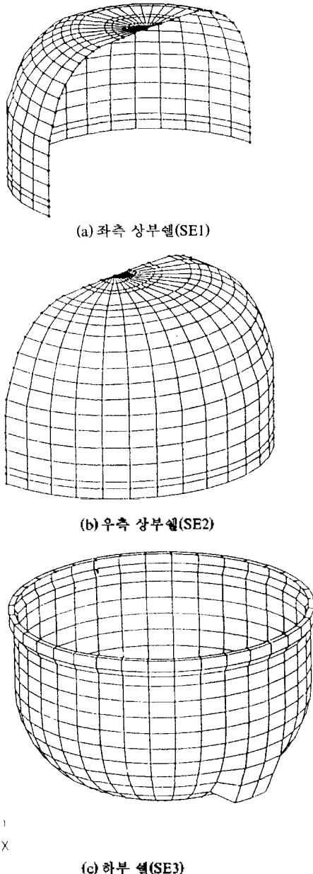
그림 5. 각 요소의 유한 요소 모델
