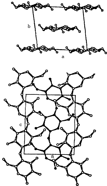
그림 3. 셀룰로오스 I 결정단위포의 모식도(평행쇄, Gardner & Blackwell).
