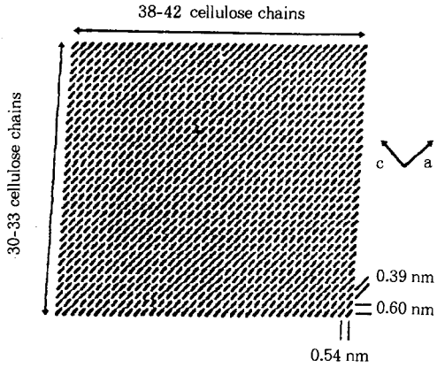
그림 16. 셀룰로오스 결정의 격자상에서 얻은 셀룰로오스 microfibril의 횡단면 모델(Sugiyama 등, 1985).
