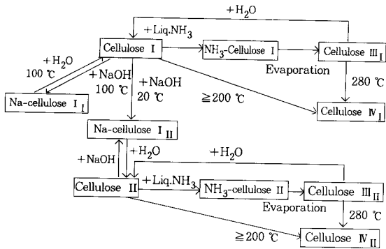
그림 6. 셀룰로오스 결정형의 변태과정.
