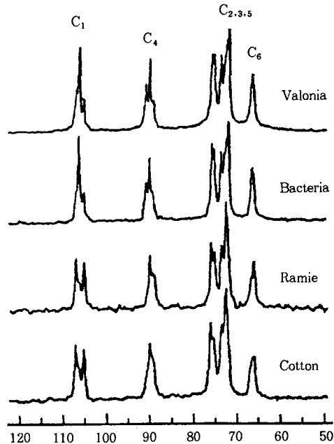
그림 5. 셀룰로오스의 CP-MAS 13 C NMR 스펙트럼.
