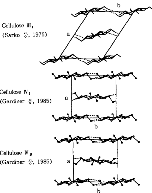
그림 10. 셀룰로오스 III, IV 결정단위포의 모식도.
