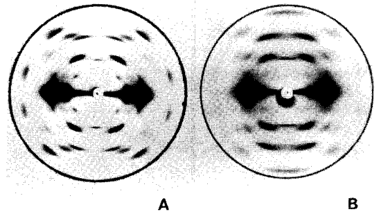
그림 7. 셀룰로오스 I(A)과 셀룰로오스 II(B)의 X선회절도.
