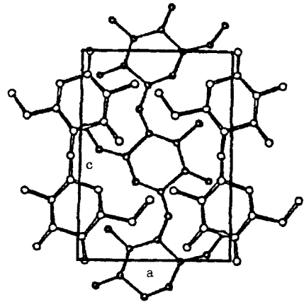
그림 8. 셀룰로오스 II 결정단위포의 모식도(Kolpak & Blackwell).
