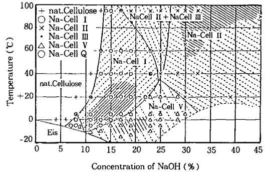
그림 11. 알칼리처리 온도 및 알칼리 농도와 Na-셀룰로오스의 형성(Sobue 등, 1939).
