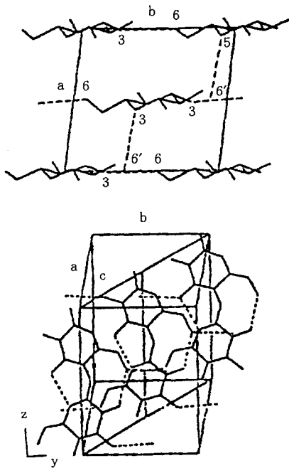
그림 4. 셀룰로오스 I 결정단위포의 모식도(평행쇄, Sarko & Muggli).
