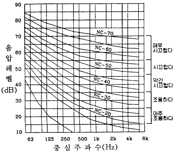
그림 1 NC곡선에 따른 소음기준치
