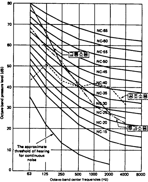
그림 4 NC35를 기준으로 한 실내소음 영향도 그래프
