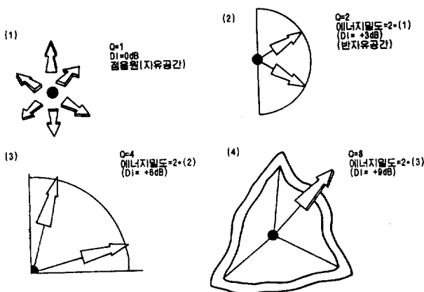
그림 3 음원의 위치별 지향지수(directivity index)
