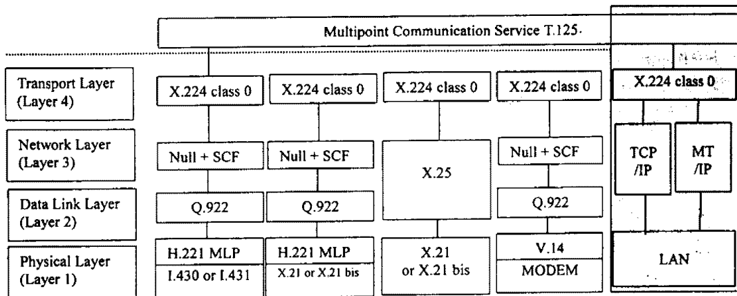
(그림 1) T.123에 정의된 프로토콜 스택과 LAN을 위한 프로토콜 (Fig. 1) Basic protocol stacks-as defined in T.123 + protocol stack for LAN
