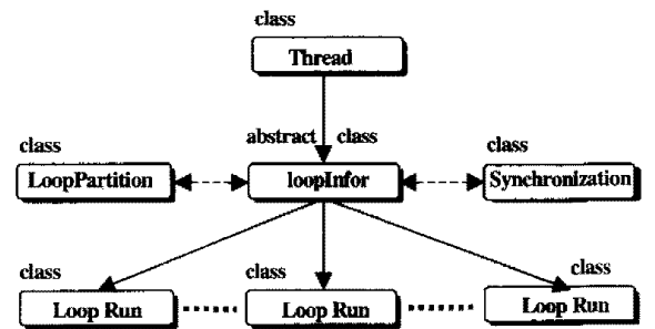
(그림 4) 클래스 계층 구조 (Fig. 4) Class Hierarchy
