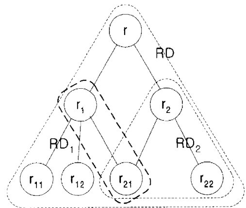
(그림 41) 직무 계층과 직무 영역 (Fig. 2) Role Hierarchy and Domain
