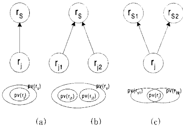
(그림 42) 직무의 기본 구성 (Fig. 3) Role Basic Organization
