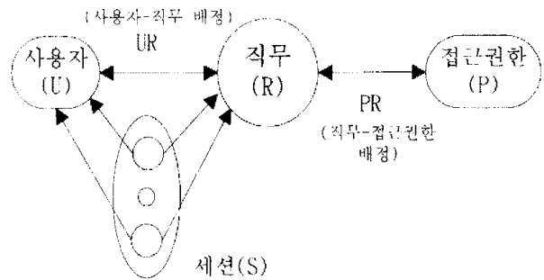
(그림 40) RBAC 모델 (Fig. 1) RBAC Model
