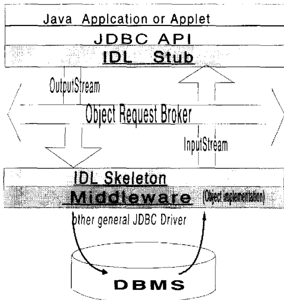
(그림 2) ORB-JDBC 하위프로토콜을 이용한 응용 시스템의 구성
