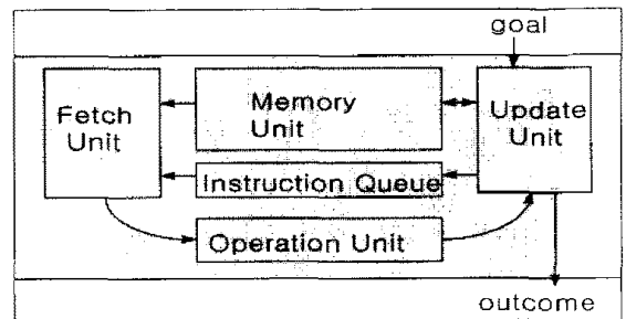
(그림 2) 인터프리터의 구조 (Fig. 2) Structure of Interpreter
