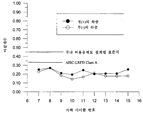
그림 9 보 이음부 마찰계수의 반복하중에 대한 거동
