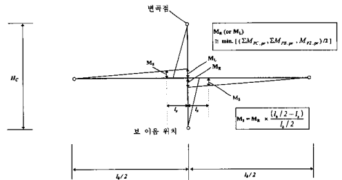
그림 11 보 이음부 검토를 위한 휨모멘트 분포
