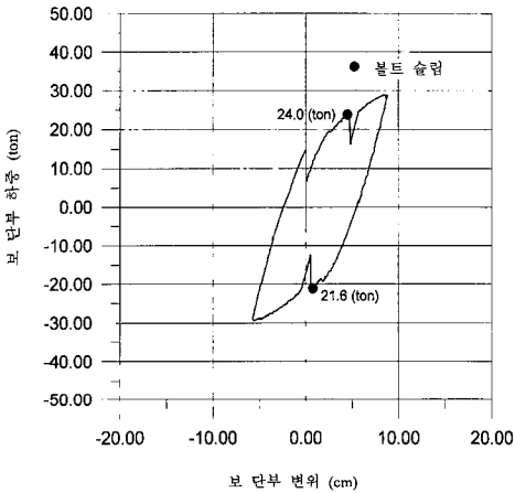
그림 6 최초 슬립 발생 때의 이력곡선 ( 4\delta_y 의 첫째 사이클)
