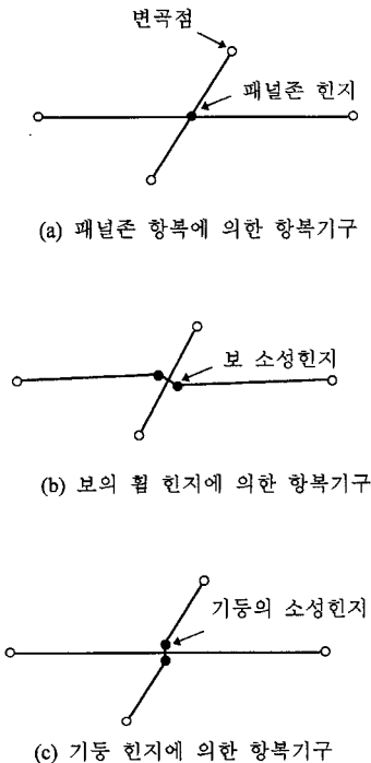
그림 10 철골 보-기둥 부분골조의 발생가능한 항복기구
