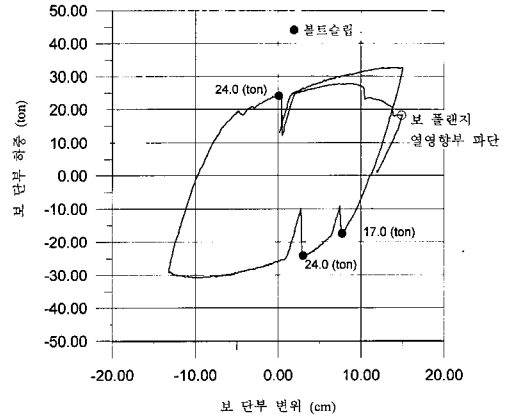
그림 7 최대 스트로크 하중에서의 이력곡선
