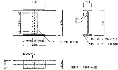
그림 5 보 이음부 상세
