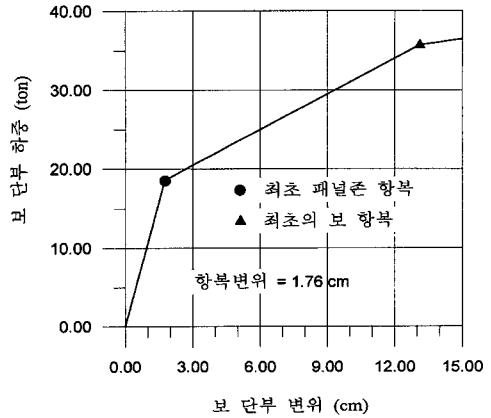
그림 4 시험체 예비해석 결과
