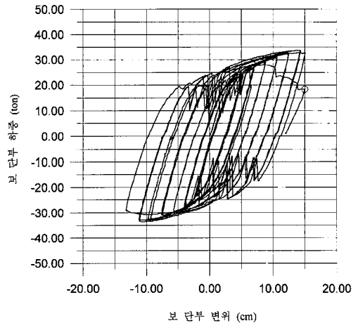
그림 8 하중 대 보 단부 변위 응답곡선
