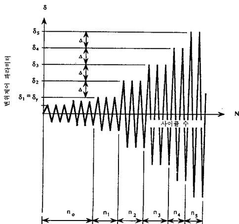
그림 3 하중이력(ATC-24)
