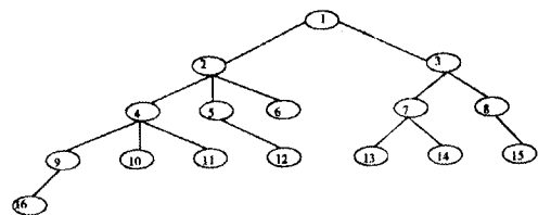
그림 2.1 초기상태 트리
