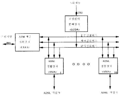
(그림 4) ADSL 가입자 정합모듈 블록도 (Fig. 4) Functional block diagram of ADSL interface module
