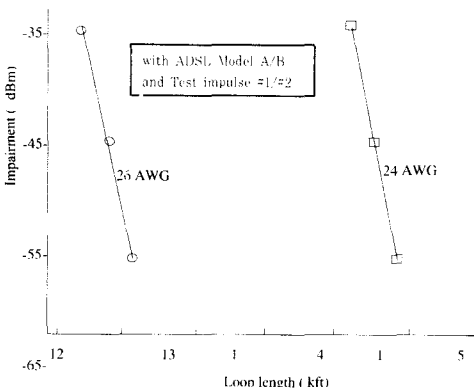
(그림 8) ADSL Model A/B 임펄스 잡음에 대한 루프 거리 성능 (Fig. 8) ADSL Model A/B and the test impulse #1/#2 vs. the loop length
