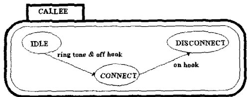
(그림 3-23) CALLEE 시스템 상태 모델 (Fig. 3-23) system state model of CALLEE
