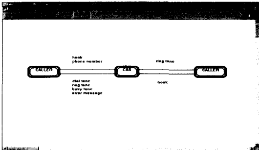
(그림 4-1) 시스템 메시지 모델 (Fig. 4-1) System message model
