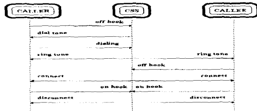
(그림 3-24) CSS 시스템 메시지 모델 (Fig. 3-24) System message model of CSS
