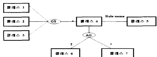
(그림 3-12) 클래스 모델 (Fig. 3-12) Class model
