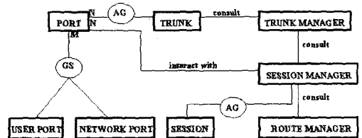
(그림 3-27) CSS 클래스 모델 (Fig. 3-27) Class model of CSS
