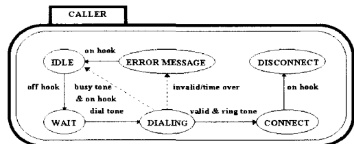
(그림 3-21) CALLER 시스템 상태 모델 (Fig. 3-21) System state model of CALLER
