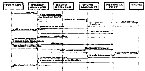
(그림 3-28) CSS 클래스 메시지 모델 (Fig. 3-28) Class message model of CSS
