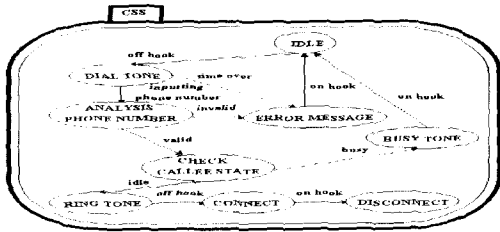
(그림 3-22) CSS 시스템 상태 모델 (Fig. 3-22) System state model of CSS
