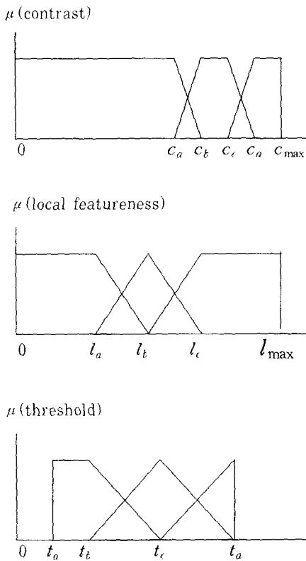
(그림 3) 입력출력 퍼지 소속함수
