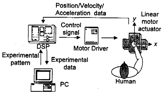
그림 2. 운동 구현기의 시스템 구성도
