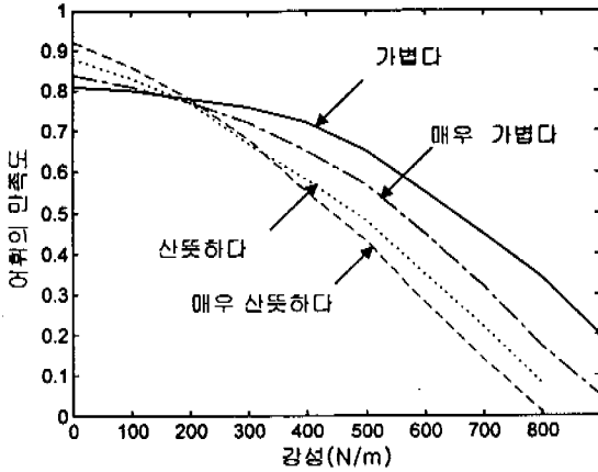
그림 8. 강성의 변화에 따른 운동감의 정량화
