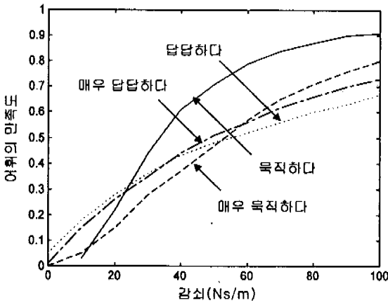
그림 9. 감쇠의 변화에 따른 운동감의 정량화
