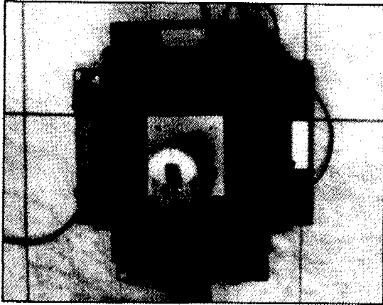
그림 1. 리니어 모터를 이용한 2차원 운동 구현기
