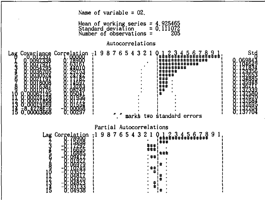
그림 1. 시차자료의 자기상관함수와 부분자기상관함수
