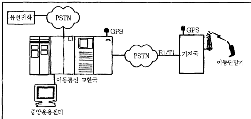
(그림 1) CDMA방식 移動통신 시스템 구성도
