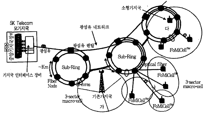
(그림 5) SK 텔레콤의 FoMiCell™(Fiber-optic Micro-Cellular)시스템
