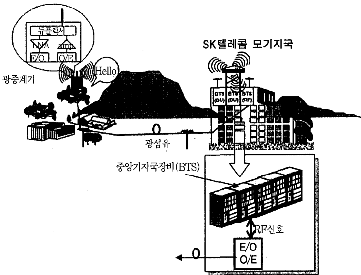
(그림 4) 전파 음영지역을 해소하기 위한 광중계기 적용예
