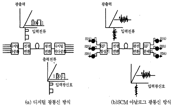
(그림 3) 디지털 광통신 방식과 SCM 아날로그 광통신 방식
