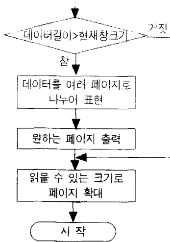
(그림 3) 순서도 (Fig. 3) Flowchart
