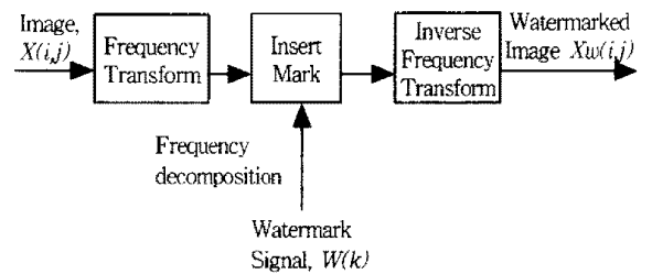
(그림 2) 주파수 영역에서의 워터마킹 삽입 알고리즘 (Fig. 2) Embedding Procedure of the watermark in the Frequency Domain
