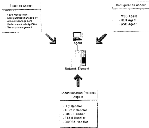
(그림 2) TMN 에이전트의 관찰측면
