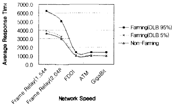
(그림 5) 전체 트랜잭션 처리시의 평균 응답시간
