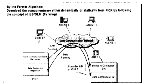
(그림 1) Farming 방법론에 의한 PCN TMN 시스템의 설계 및 구현
