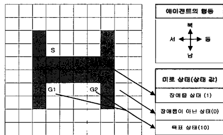
(그림 9) 미로 환경
