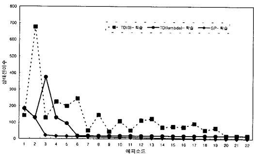
(그림 11) G2 상태에 대한 학습 결과
