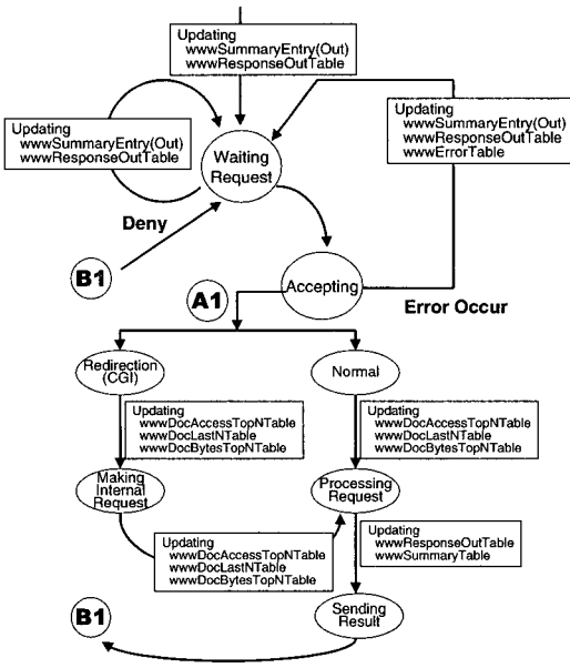
(그림 4) WWW Service의 요청 처리
