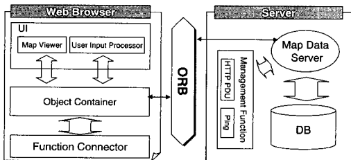
(그림 2) Map Editor의 구조
