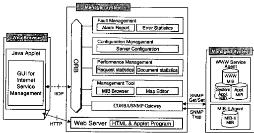
(그림 1) 인터넷 서비스 관리 시스템의 구조
