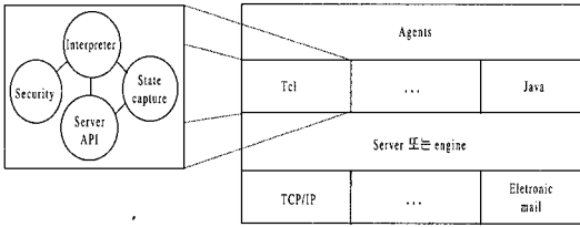
(그림 4) AgentTcl의 구조
