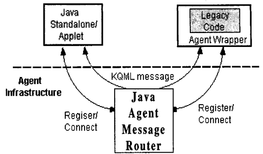
(그림 2) 자바 에이전트 라우터의 동작의 예
