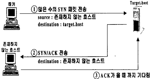
(그림 7) SYN flooding
