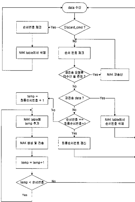
그림 3. 수신단 동작절차
