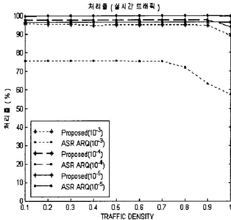
그림 5. 실시간 트래픽의 처리율
