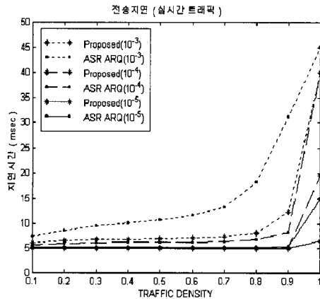
그림 4. 실시간 트래픽의 전송지연
