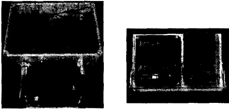
그림 7. 설계된 마이크로파 무선인식시스템 (a) 질문기 (b) 응답기
