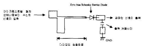
그림 6. 검파기의 구조
