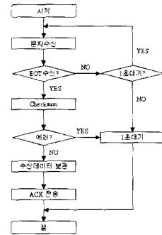
그림 9-a. 응답기의 데이터 전송흐름도
