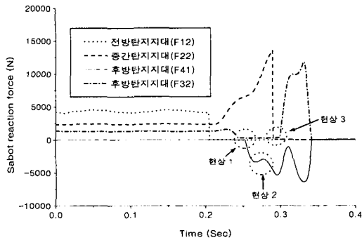
[그림 11] 탄지지대 반력 (간극 3)
