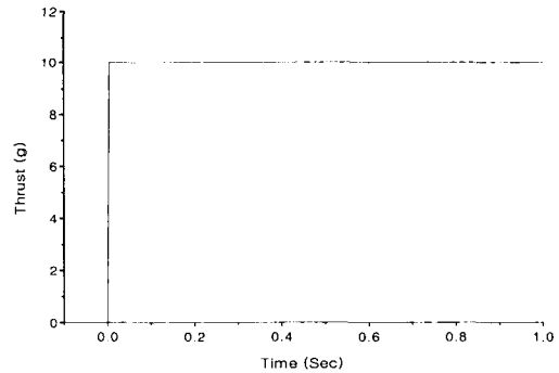
그림 5 유도탄 추력 모델링
