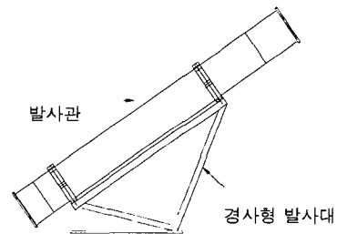
그림 1 발사대 형상
