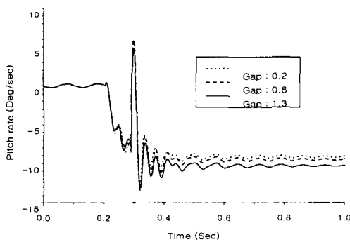
[그림 12] 유도탄 피치 각속도 (탄지지대 강성 5000 N/mm)
