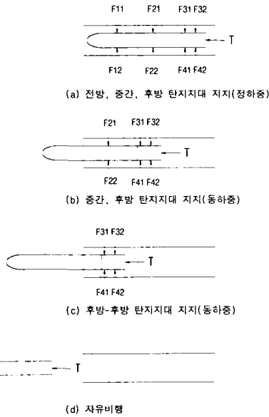
그림 3 유도탄 초기 발사단계
