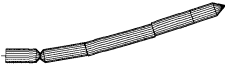
(그림 6) 유도탄 1차 모드 (3.528Hz)
