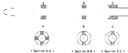
그림 2 유도탄과 발사관의 조립형상
