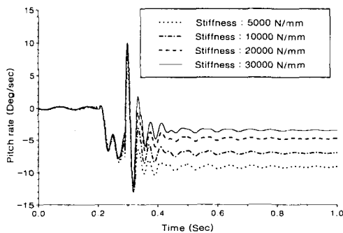
그림 14 탄지지대 강성에 따른 피치각속도 변화
