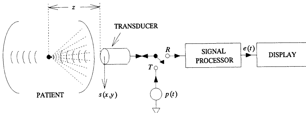
Fig. 1 초음파 영상진단장치의 block diagram
