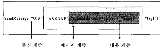
(그림 6) 계층화된 구조의 통신 명령
