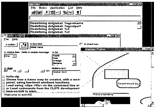
(그림 8) INAS 버전 2의 그래픽 사용자 인터페이스 구축 기능의 예
