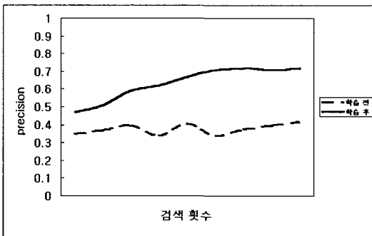
(b) 정확률(precision)의 비교
