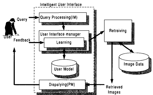
(그림 1) 검색 시스템에서의 지능 사용자 인터페이스의 역할
