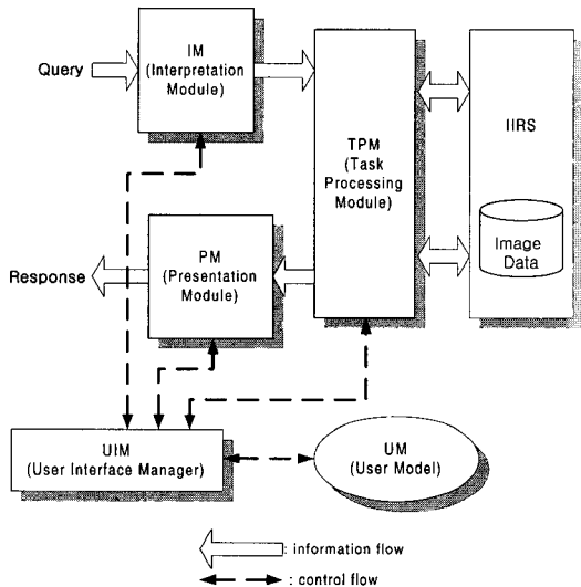
(그림 3) UII 개념모델
