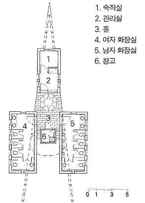
1층평면도
