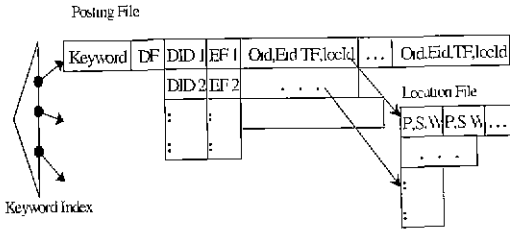
(그림 10) Keyword 인덱스의 구조
