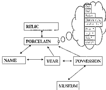
(그림 8) 구성된 트리의 각 엘리먼트의 구조정보
