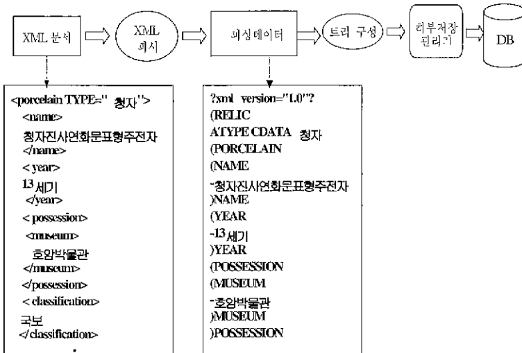
(그림 7) XML 문서의 파싱과 트리 구성 과정
