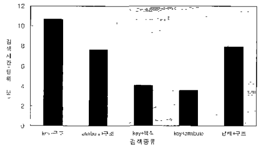
(그림 19) 복합질의의 검색시간
