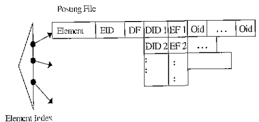
(그림 12) 엘리먼트 인덱스의 구조
