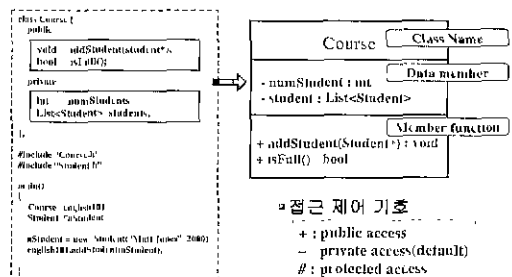
(그림 1) 클래스 다이어그램의 예
