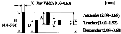
(그림 2) 우편용 4-state 바코드 인쇄규격
