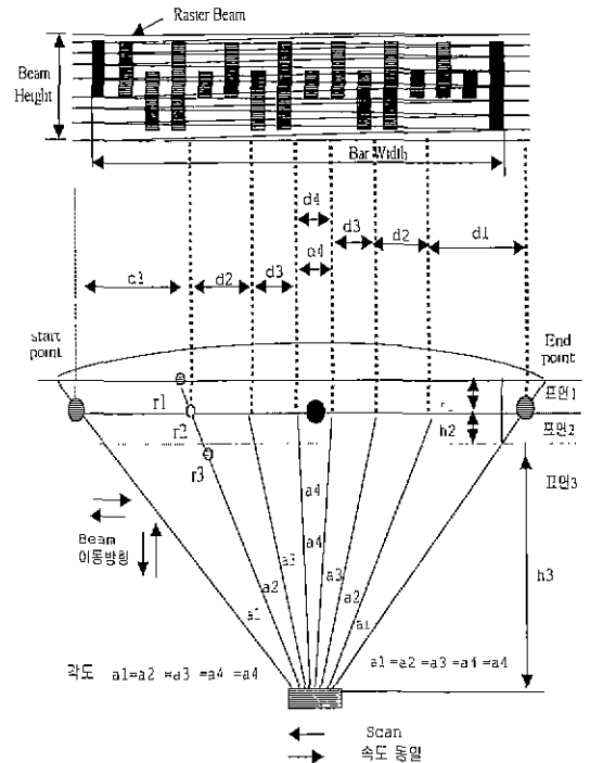
(그림 4) Raster beam의 주사방법
