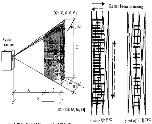
4개의 중심 축에 의한 beam의 이동 방향 - 상에서 하로 beam의 이동 방향 a0, b1, a2, b3 - 하에서 상으로 beam의 이동 방향 b3, b2, a1, b0
