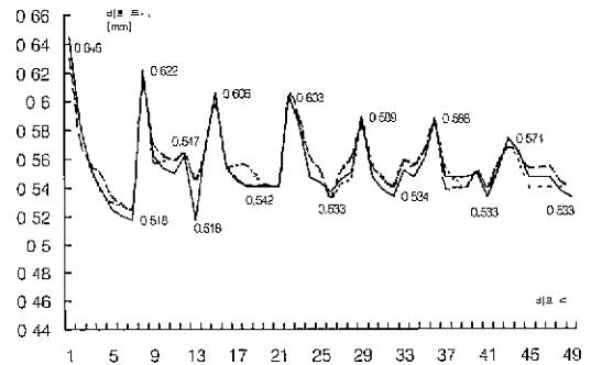
(그림 9) 판독오차 범위 값의 시험 (광원과의 거리 120mm, 3회)
