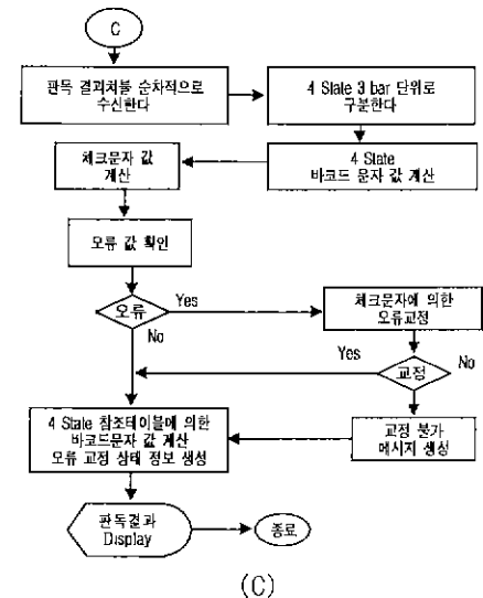
(그림 8) 4-state 바코드판독기의 판독 절차
