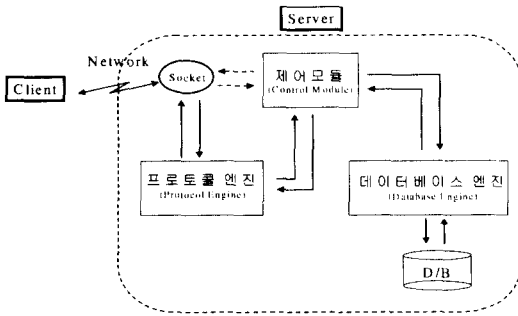
(그림 1) 기본적인 Z39.50 서버의 구성
