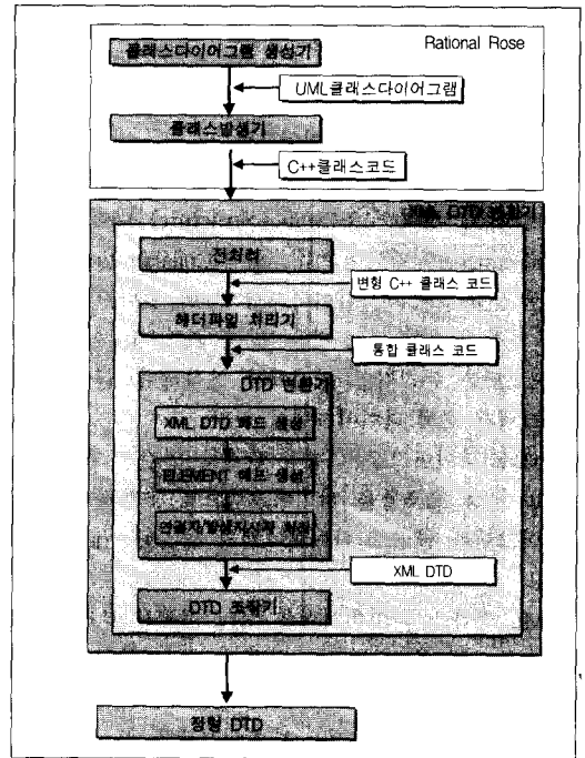
(그림 4) 시스템 구성도
