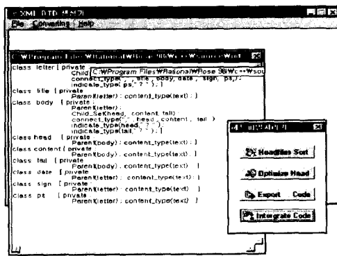
(그림 12) 통합 클래스코드 화면
