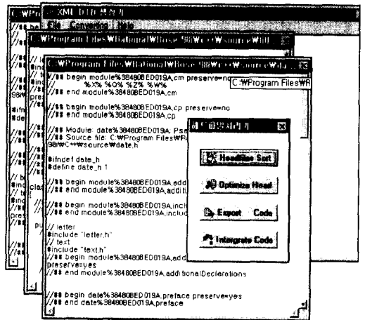
(그림 10) 헤더파일 처리기 화면
