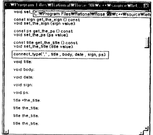
(그림 9) 관계성이 첨가된 헤더파일
