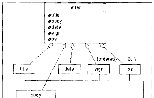
(그림 6) 관계성이 포함된 클래스 다이어그램
