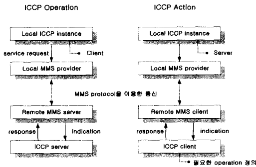
(그림 7) ICCP의 동작과정
