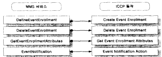
(그림 4) MMS와 ICCP에서 이벤트 서비스 비교
