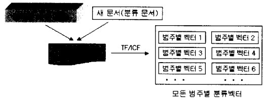
(그림 5) 분류 벡터 생성과정
