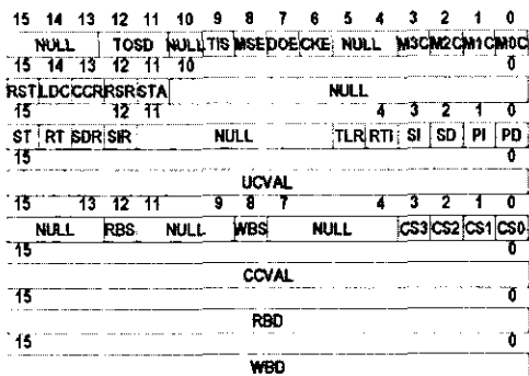
그림 7. 내부 레지스터 각 비트의 기능
