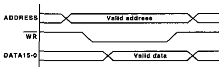
그림 5. 프로세서의 쓰기 타이밍 다이어그램
