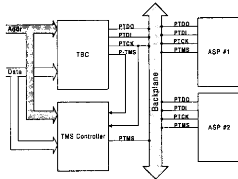
그림 1. ASP(Addressable Scan Port)를 이용한 시스템 레벨의 테스트
