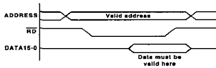
그림 6. 프로세서의 읽기 타이밍 다이어그램
