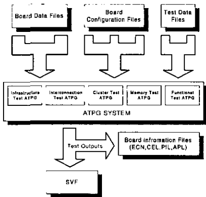
그림 13. ATPG툴의 블록 다이어그램
