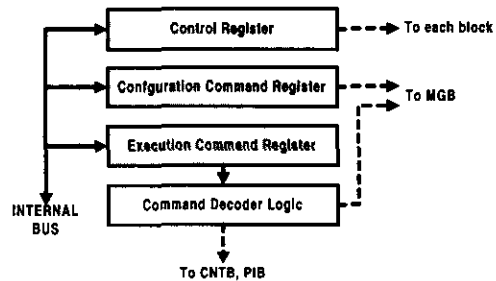
그림 9. 제어 및 명령 블록
