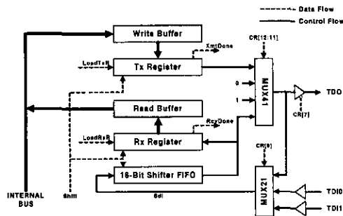
그림 11. 직렬 데이터 송수신 블록
