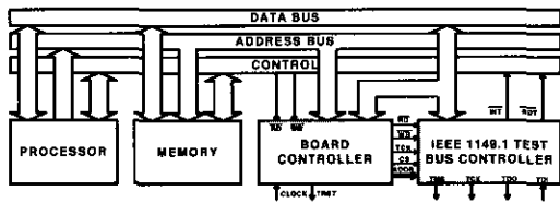
그림 4. 프로세서 인터페이스
