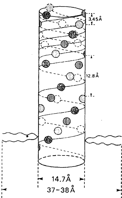
그림 9. (LP 2 , LU 2 ) n 수소결합 고분자들이 자기조립을 통해 형성되는 삼중나선구조를 갖는 원기둥 초분자구조.
