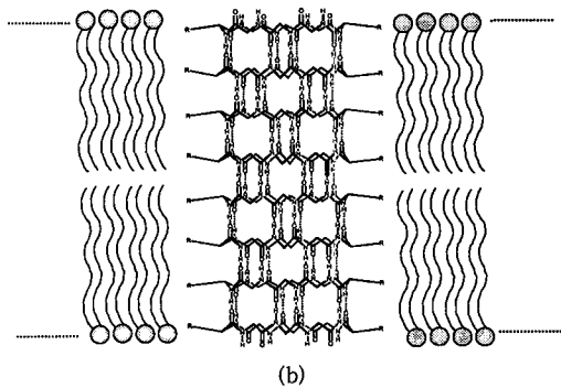
그림 10. (a) 평평한 링 형태의 구조를 갖는 펩티드 기본단위의 화학구조 (D 또는 L : 아미노산의 키랄성질). (b) 이중 지질막 안에서 펩티드 기본단위들이 자기조립을 통해 형성되어지는 튜브구조.
