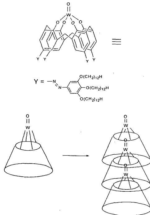
그림 3. 칼리스 아렌 유도체에 의해 형성된 원기둥형 초분자구조.
