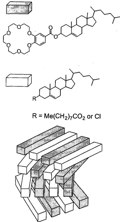
그림 4. 크라운 에테르를 함유한 콜레스테릭 유도체의 키랄 네마틱 구조.
