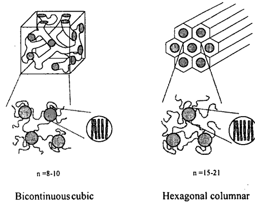
그림 7. 수소결합 주사슬 고분자의 코일길이 변화에 따른 초분자구조의 조절.
