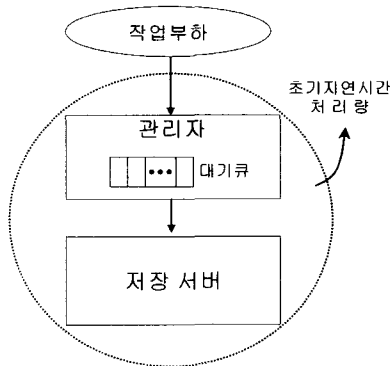
(그림 6) 시뮬레이터의 구성
