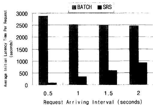
(그림 7) 정책에 따른 초기지연시간
