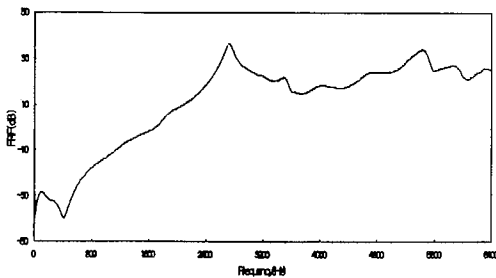
Fig. 11 FRF of top cap
