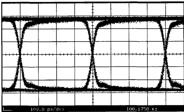
그림 6. 송신된 2.5 Gbps 광신호의 Eye Diagram.
