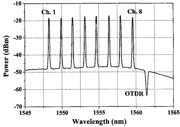
그림 5. WDM 8 채널 전송 결과(RBW = 0.2 nm).
