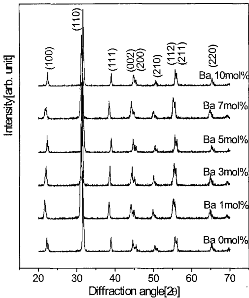
그림 2 Ba 치환에 따른 X-선 회절 모양 Fig. 2 X-Ray diffraction patterns with the substitution of Ba
