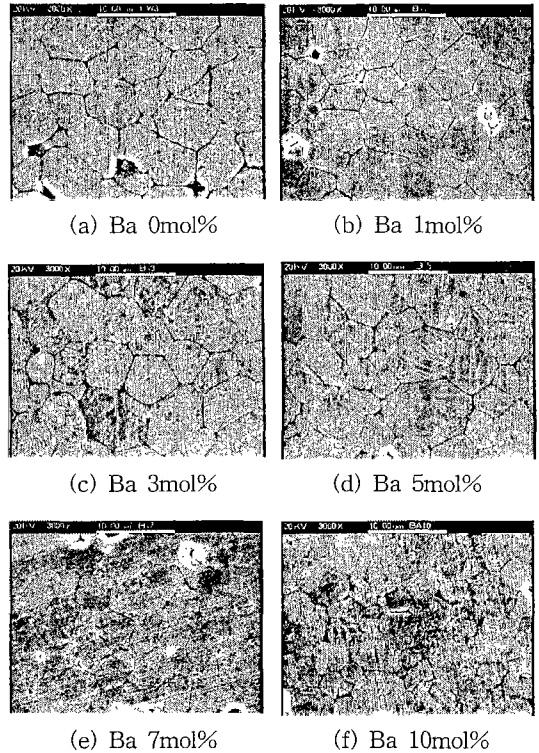
그림 3 Ba 치환에 따른 미세구조(SEM)
