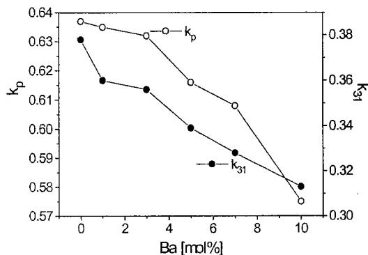
그림 6 Ba 치환에 따른 전기기계결합계수( k_p , k_{31} )
