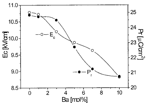
그림 5 Ba 치환에 따른 항전계와 잔류분극
