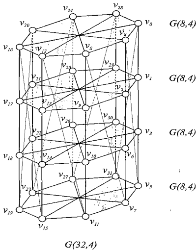
그림 2 G(32,4) 의 재귀적 구조
