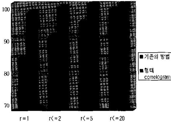
(그림 9) 회전 변화에 대한 검색률 비교
