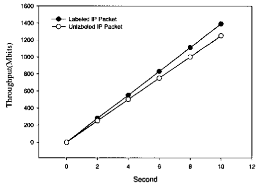
그림 4. Case of 150 Mbit/s
