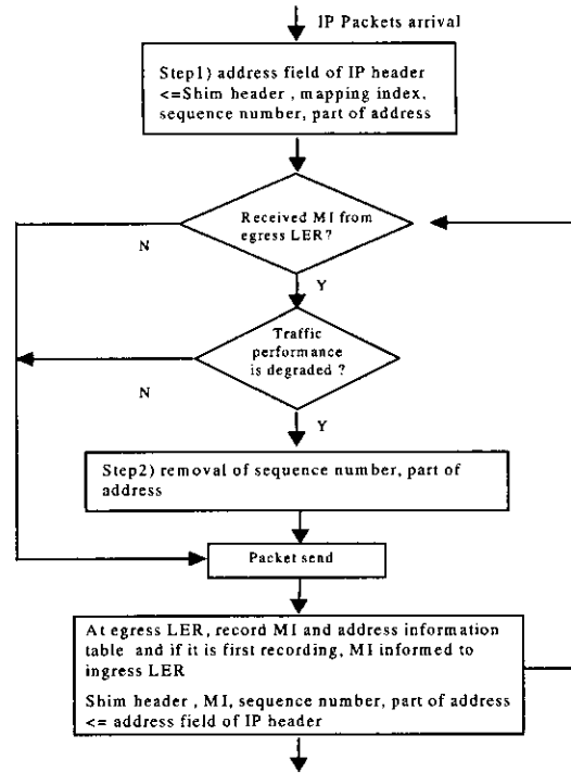
그림 10. Proposed MPLS shim header allocation algorithm
