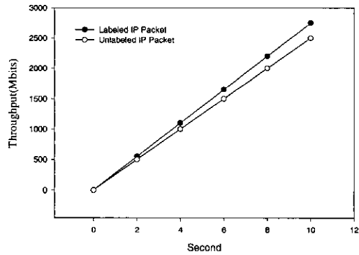
그림 5. Case of 300 Mbit/s
