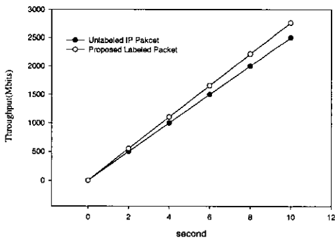
그림 12. Case of 300 Mbit/s
