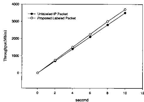
그림 13. Case of 450 Mbit/s
