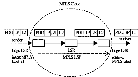
그림 2. MPLS packet flow
