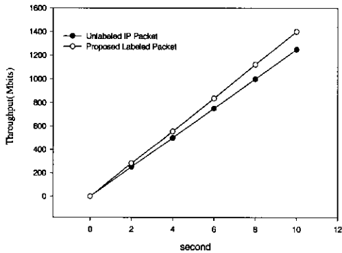
그림 11. Case of 150 Mbit/s
