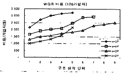
(a) WGR 비용/가입자
