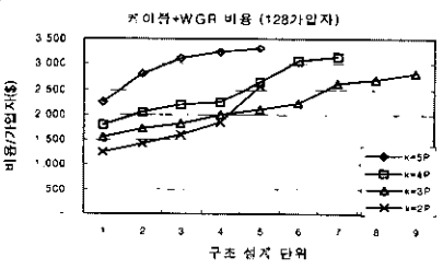
(c) WGR 및 케이블 비용/가입자
