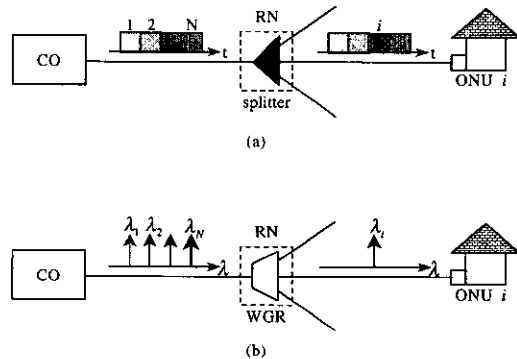
그림 1. TDM-PON과 WDM-PON의 비교 (a) TDM-PON 방식 (b) WDM-PON 방식
