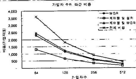
그림 9. 가입자수에 따른 광 가입자망의 구성 비용
