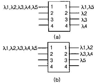
그림 2. M=4인 WGR의 파장 라우팅 (a)C=1, (b)C=2
