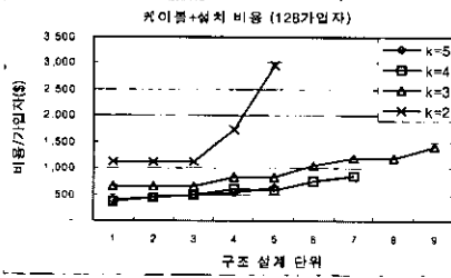
(b) 케이블 및 설치 비용/가입자
