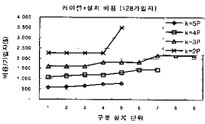
(b) 케이블 및 설치 비용/가입자
