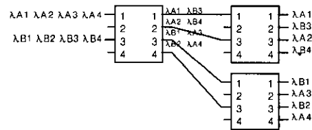
그림 4. 다중 성형 광 가입자망의 구성 예
