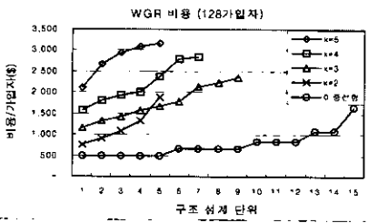
(a) WGR 비용/가입자
