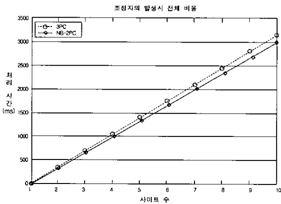
(그림 6) 조정자 고장 발생 시 완료규약 비용
