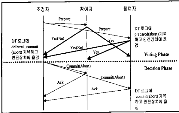
(그림 1) NB-2PC 규약
